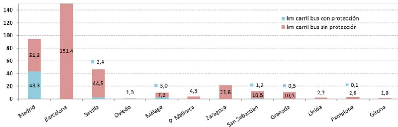
Figura 19 - Carriles bus en la ciudad capital. Año 2013
