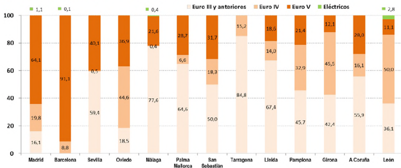
Figura 16 – Autobuses urbanos por tecnología de motor respecto al total de la flota (en %). Año 2013
