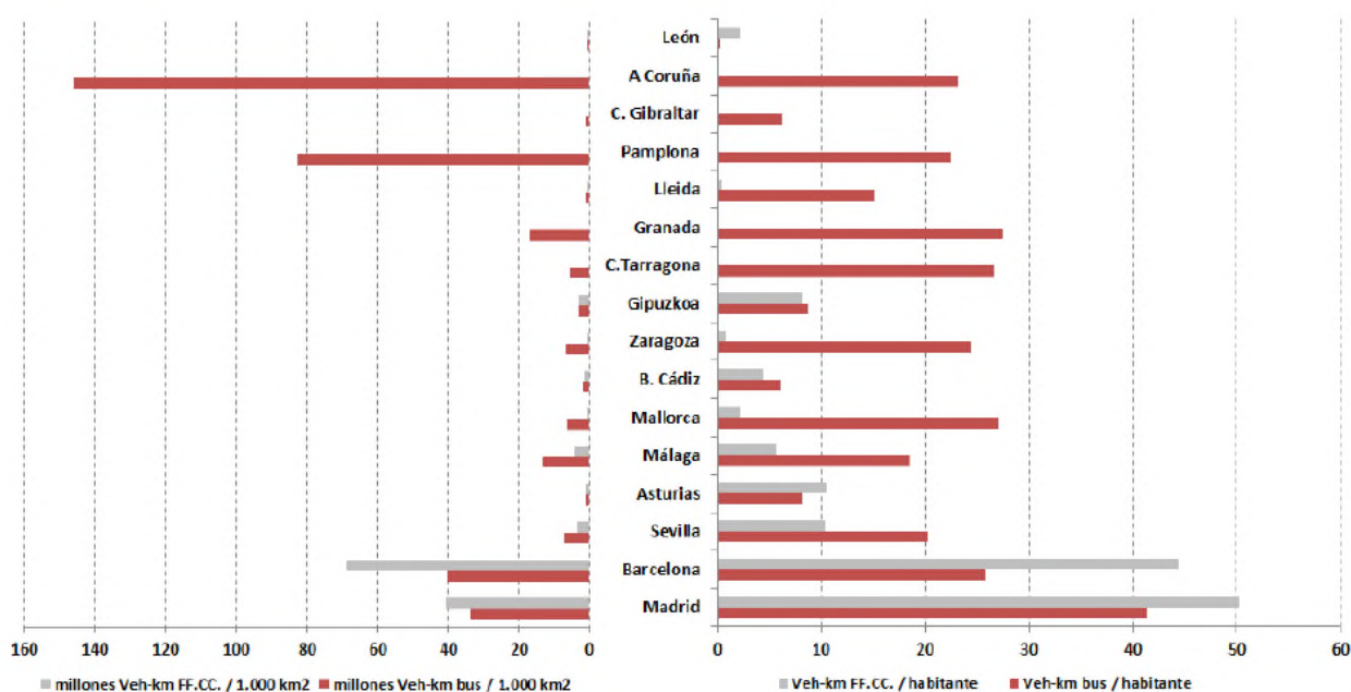
Figura 13 - Densidad de vehículos-km ofertados, por población y superficie. Año 2013
